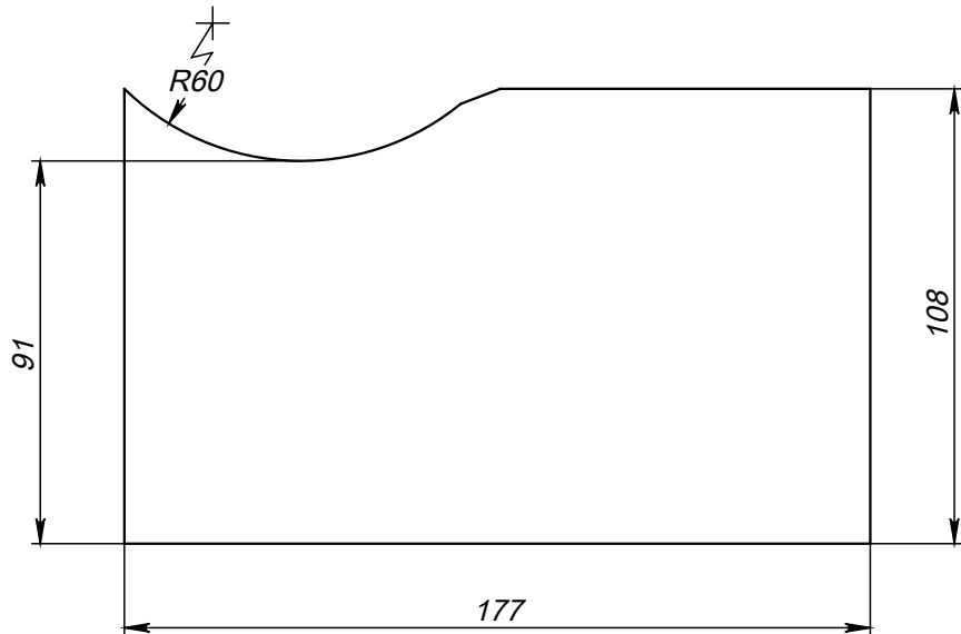
Поз.3 (Угольник)
